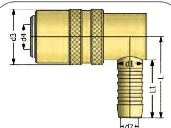
Standard hose tail socket 90° Kupplung mit 90° Standard-Schlauchtülle
