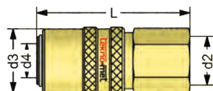
Parallel Female Thread Kupplung mit Innengewinde
