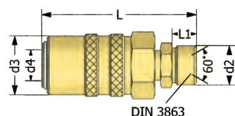
Parallel Male Thread Kupplung mit Aussengewinde
