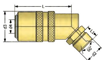
Cylindrical Male Thread socket 45° Kupplung mit 45° Aussengewinde zylindrisch
