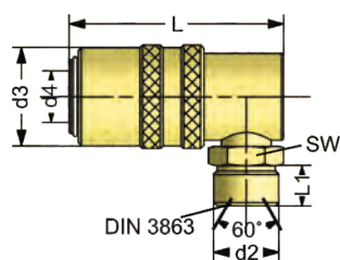
Cylindrical Male Thread socket 90° Kupplung mit 90° Aussengewinde zylindrisch
