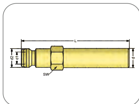
Steel Extension Tube Verlängerunsnippel aus Stahl
