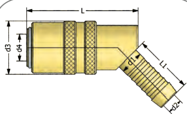
Standard hose tail socket 45° Kupplung mit 45° Standard-Schlauchtülle
