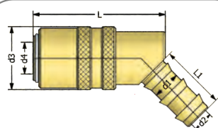
Push-Lock hose tail socket 45° Kupplung mit 45° Schnellsteck-Schlauchtülle
