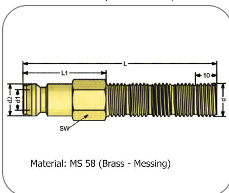
Extension plug without thread Verlängerunsnippel ohne Gewinde
