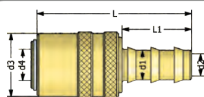
Push-Lock hose tail socket Kupplung mit gerader Schnellsteck-Schlauchtülle
