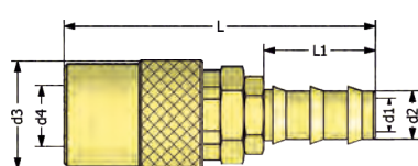
Push-Lock hose tail socket Kupplung mit gerade Schnellsteck-Schlauchtülle
