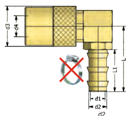
Standard hose tail socket 90° Kupplung mit 90° Schnellsteck-Schlauchtülle
