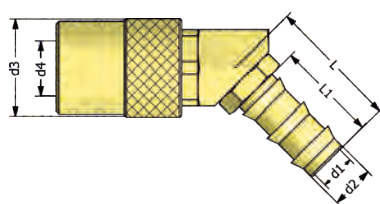
Push-Lock hose tail socket 45° Kupplung mit 45° Schnellsteck-Schlauchtülle
